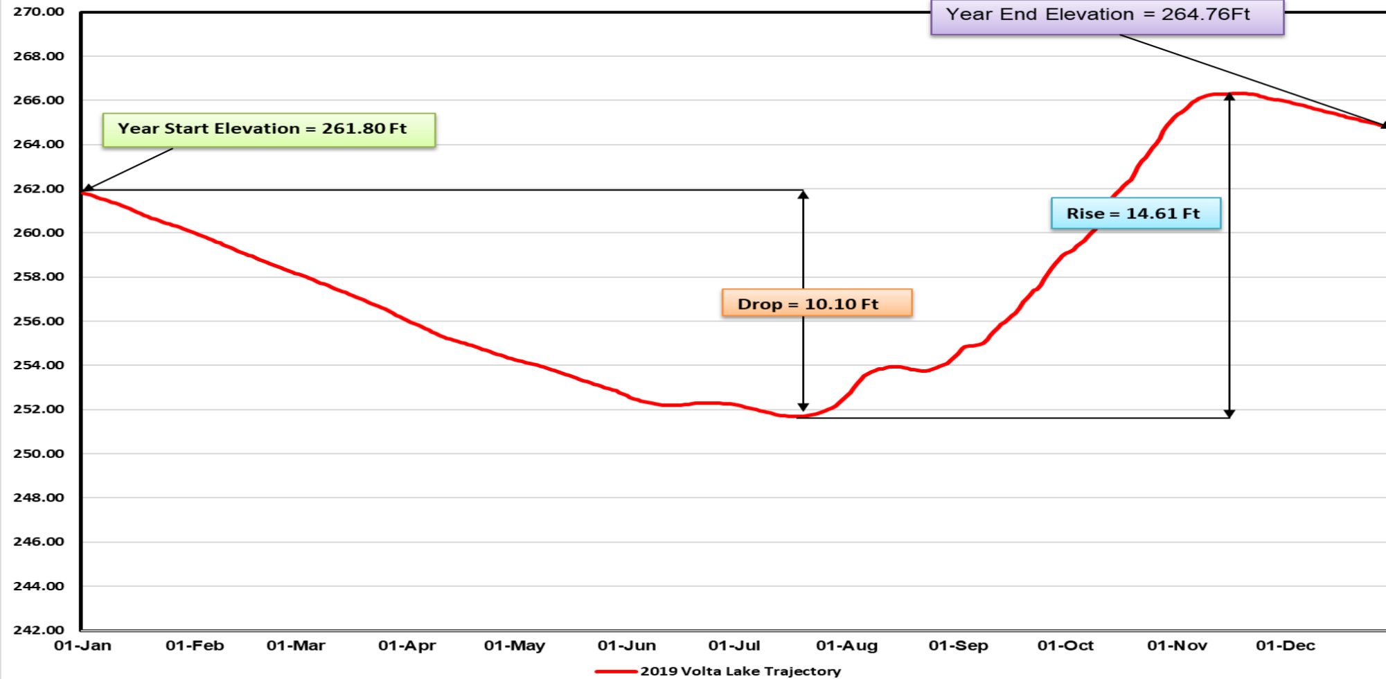
2019 VOLTA LAKE TRAJECTORY
